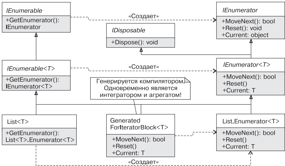
Рис. 4.3. Обобщенные и необобщенные итераторы
