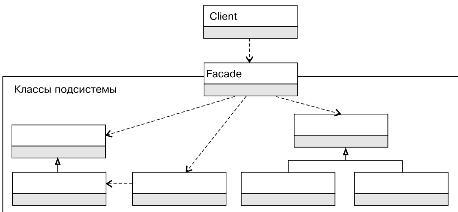
Рис. 13.2. Классическая диаграмма классов паттерна Фасад
