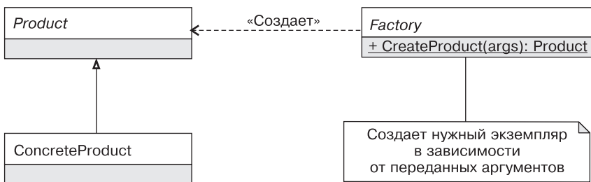
Рис. 10.2. Диаграмма статического фабричного метода
