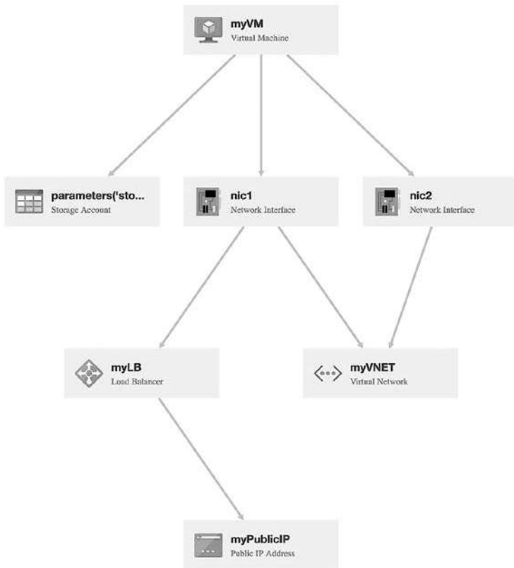
Рис. 6.9. Наглядное представление ресурсов, описанных шаблоном ARM
