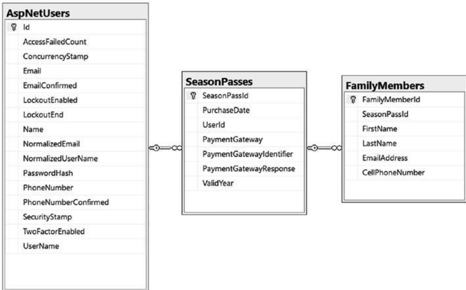
Рис. 3.1. Структура таблиц, которые могут использоваться для моделирования приобретения сезонных абонементов
