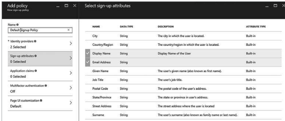
Рис. 13.4. Настройка регистрационной политики по умолчанию для каталога
