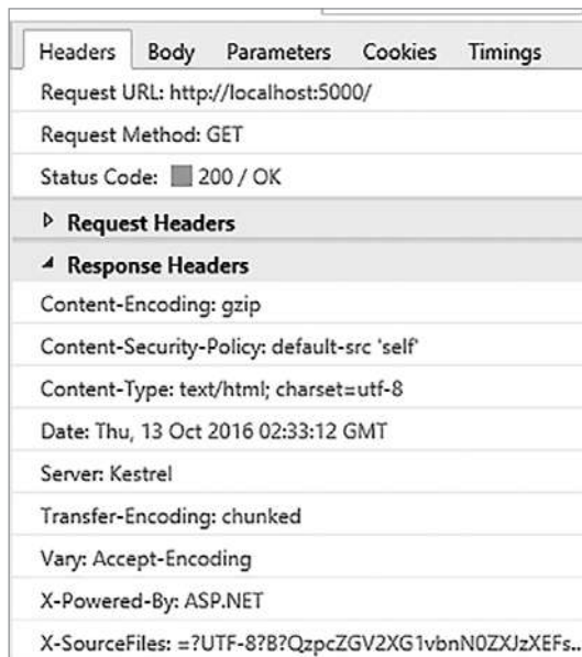
Рис. 21.3. Заголовок ответа Content-Security-Policy
