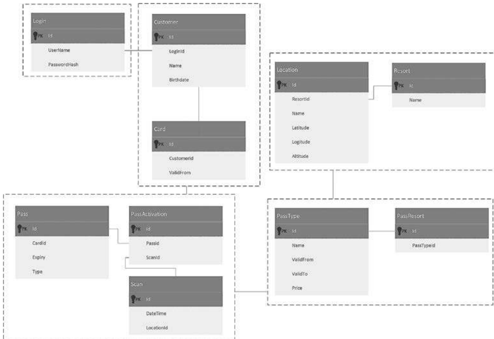
Рис. 4.2. Диаграмма отношений между сущностями с разбиением на ограниченные контексты
