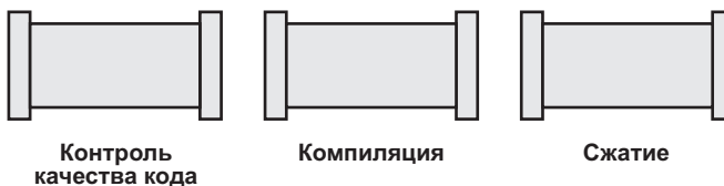
Рис. 15.3. Конвейер сборки
