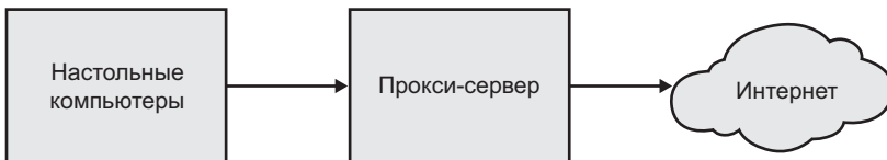
Рис. 6.1. Прокси-сервер
