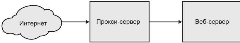
Рис. 6.2. Обратный прокси-сервер
