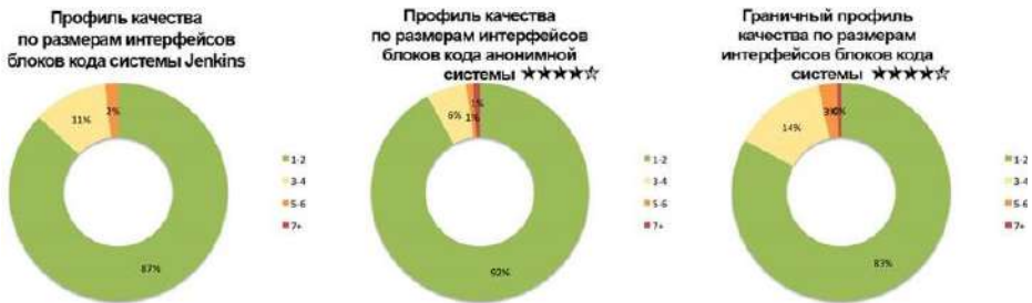
Рис. 5.1 ❖ Три профиля качества по размерам интерфейсов блоков кода
