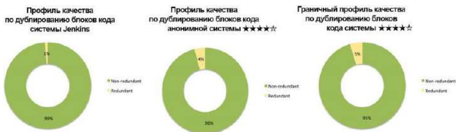
Рис. 4.1 ❖ Три профиля качества по дублированию кода
